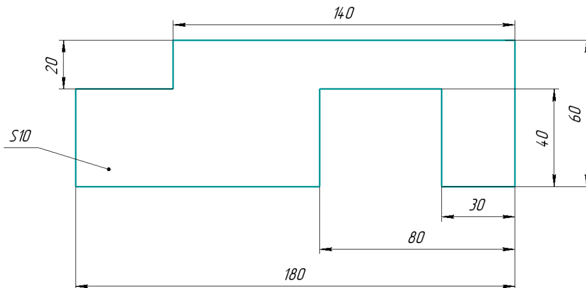
Чертёж детали
