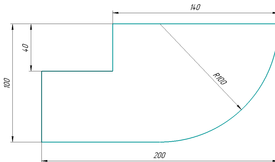
Чертёж детали
