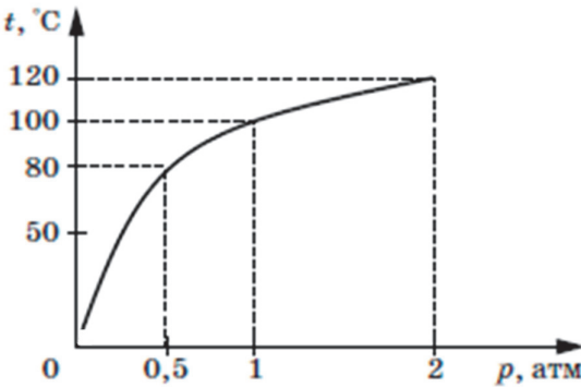
Рисунок 1. Зависимость температуры кипения воды от давления
