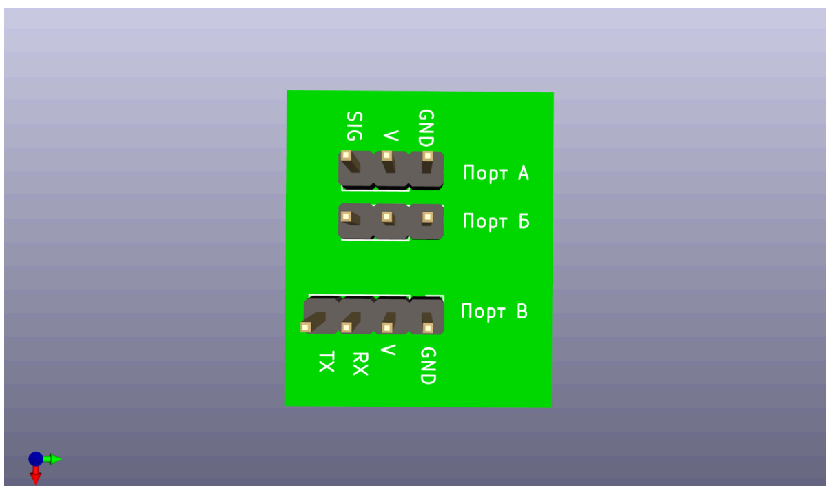
Рис 1. Возможный вид разъемов, расположенных на устройстве
