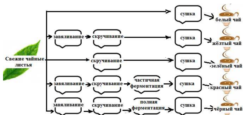
Технологическая схема переработки чая
